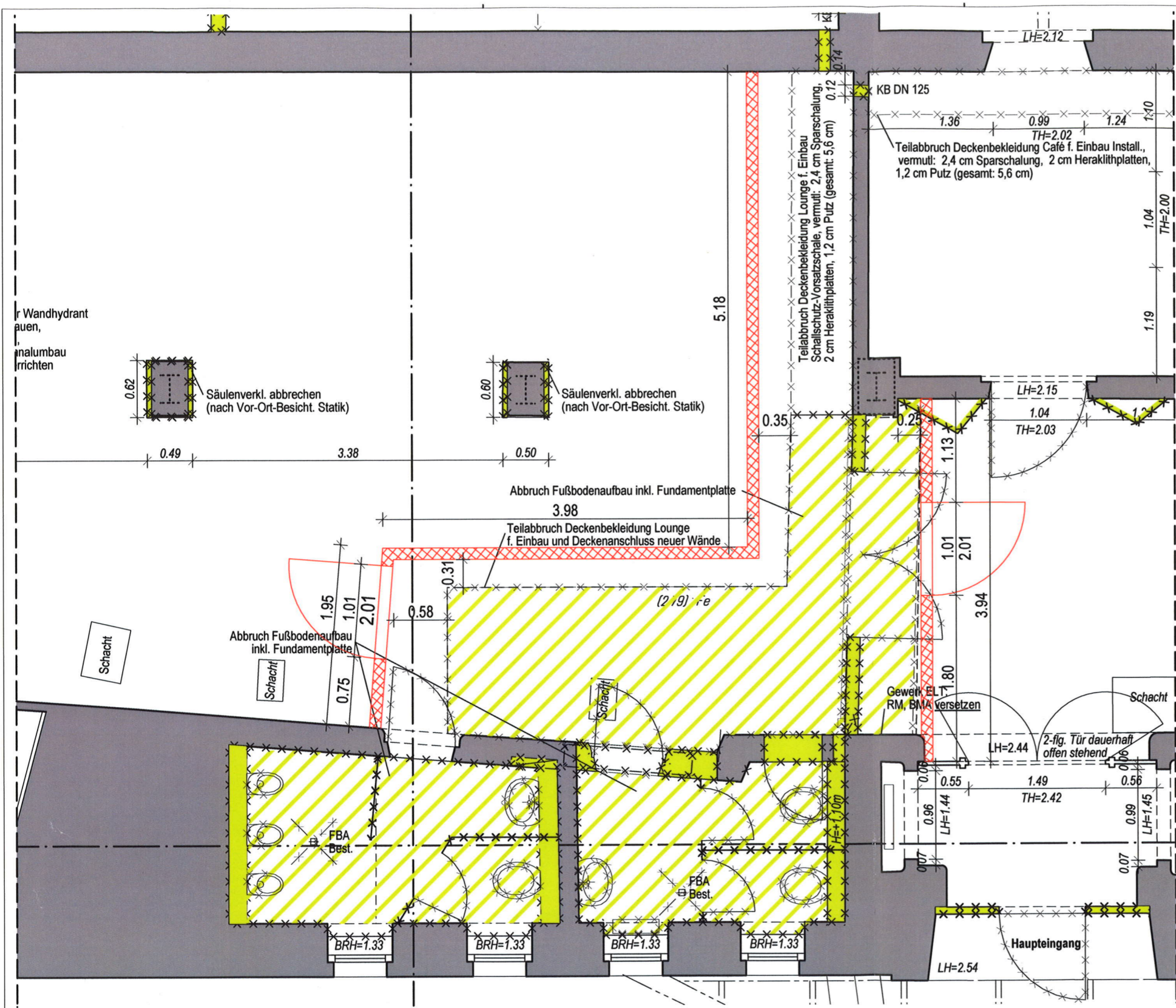
Skizze Staubschutz für Umbau WCs Lounge (Grundrissausschnitt EG) M 1:50
